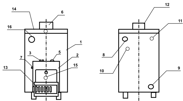
Рис. 1. Устройство котла
