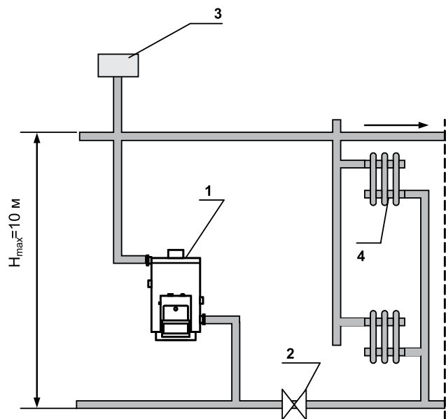
Рис. 2. Схема монтажа системы отопления
